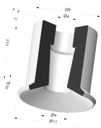
Flachsauggreifer Serie 9 Ø 11MM
