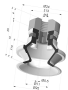
Sauggreifer 1.5 Falten Serie 91 Ø 22.2MM
