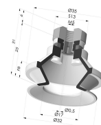
Sauggreifer 1.5 Falten Serie 91 Ø 31.8MM
