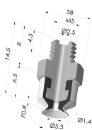
Flachsauggreifer Serie PFTM Ø 5.3 mm
