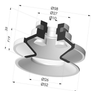
Sauggreifer 1.5 Falten Serie 91 Ø 50MM
