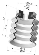
Sauggreifer 4.5 Falten Serie 92 Ø 20MM
