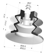
Sauggreifer 2.5 Falten Serie 96 Ø 52MM
