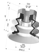
Ventosa 2.5 Fuelles Serie 96C Ø 50MM
