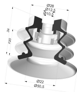
Ventosa 2.5 Fuelles Serie 96C Ø 50MM
