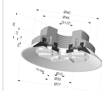
Ventosa Plana Serie 90 Ø 75MM
