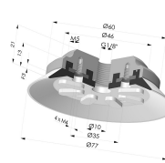
Ventosa Plana Serie 90 Ø 75MM
