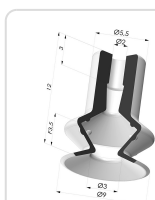
Ventosa 1.5 Fuelles Serie 91 Ø 9,2MM
