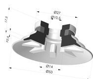
Ventosa Plana Serie 90 Ø 53MM
