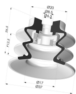
Ventosa 2.5 Fuelles Serie 96 Ø 35MM
