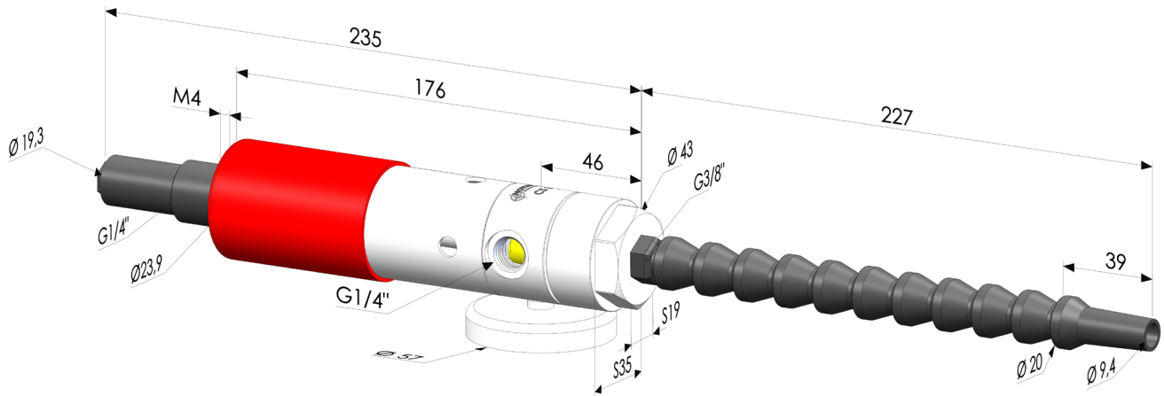
PISTOLETS À AIR FROID CSI0-R
