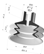
Ventouse 2.5 Soufflets Série 8 Ø53MM
