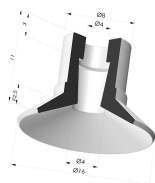
Ventouse Plate Série 9 Ø 16MM Référence produit : 9 16-- A
