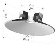
Ventouse Plate Série 9 Ø 31.5MM
