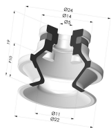
Ventouse 1.5 Soufflets Série 91 Ø 22,2MM
