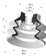
Ventouse 2.5 Soufflets Série 96C Ø 20MM
