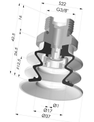
Ventouse 2.5 Soufflets Série 96 Ø 35MM
