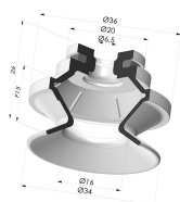
Ventouse 1.5 Soufflets Série 91 Ø 34MM
