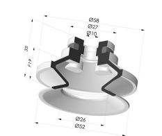
Ventouse 1.5 Soufflets Série 91 Ø 50MM Référence produit : 91 50-- A
