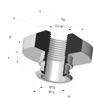
Insert Démontable Femelle 1/8G Référence produit : 9G18-2
