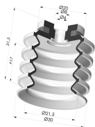
Ventouse 4.5 Soufflets Série 92 Ø 30MM
