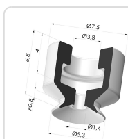
Ventosa Piatta Serie PFG Ø 5.3 mm
