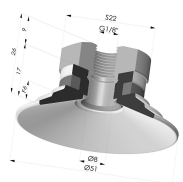
Ventosa Piatta Serie 9 Ø 51MM
