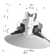
Ventosa Piatta Serie 9 Ø 51MM
