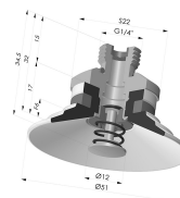
Ventosa Piatta Serie 9 Ø 51MM
