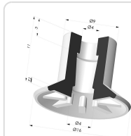
Ventosa Piatta Serie 90 Ø 16.5MM
