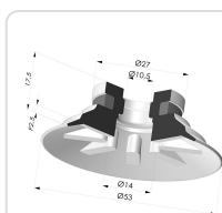
Ventosa Piatta Serie 90 Ø 53MM
