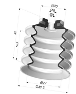
Ventosa 4.5 Soffietti Serie 92 Ø 40MM
