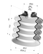
Ventosa 4.5 Soffietti Serie 92 Ø 40MM
