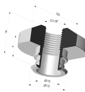
Inserto a resca Femmina G1/8"
