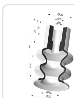
Ventosa 2.5 Fole Série 8B Ø 30MM
