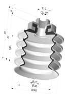
Ventosa 4.5 Fole Série 92 Ø 50MM
