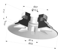
Ventosa plana Série 90 Ø 53 mm
