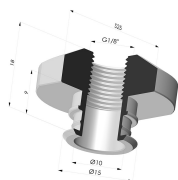
Inserto fêmea removível 1/8G
